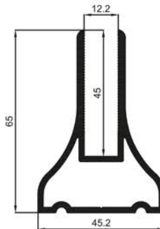
M1-12/A (7.3 kg / 6 mt) Eko Etek Profili Eco Series Bottom Profile Нижний профиль для оконных ограждений - эко بروفيل ارضي اقتصادي للزجاج
