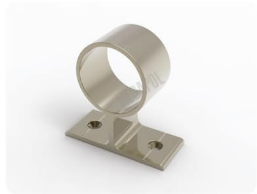
M21-07/B 40'lik Boru Yandan Ara Bağlantı 40 mm Pipe Lateral Connection Боковое крепление для 40 мм трубы وصلة جانبية لانبوب 40 مم
