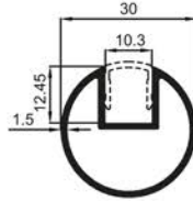
M1-11/A (3 kg / 6 mt) 30 mm Kanallı Boru 30 mm Pipe with Channel 30 мм труба с каналом بروفيل 30 مم بقناة
