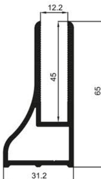
M1-12/C (6.5 kg / 6 mt) Eko Etek Profili Düz Eco Series Flat Bottom Profile Прямой Нижний профиль для оконных ограждений Эко بروفيل قاعدي للزجاج مسطح اقتصادي
