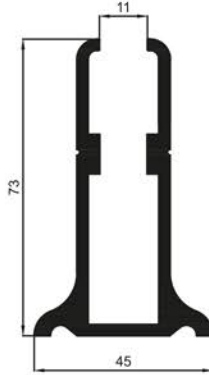
M1-12 (11.4 kg / 6 mt) Camlı Korkuluk Alt Profili Glazing Balustrade Bottom Profile Нижний профиль для оконных ограждений بروفيل سفلي للزجاج
